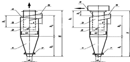
Циклон ЦН-11 без улитки
